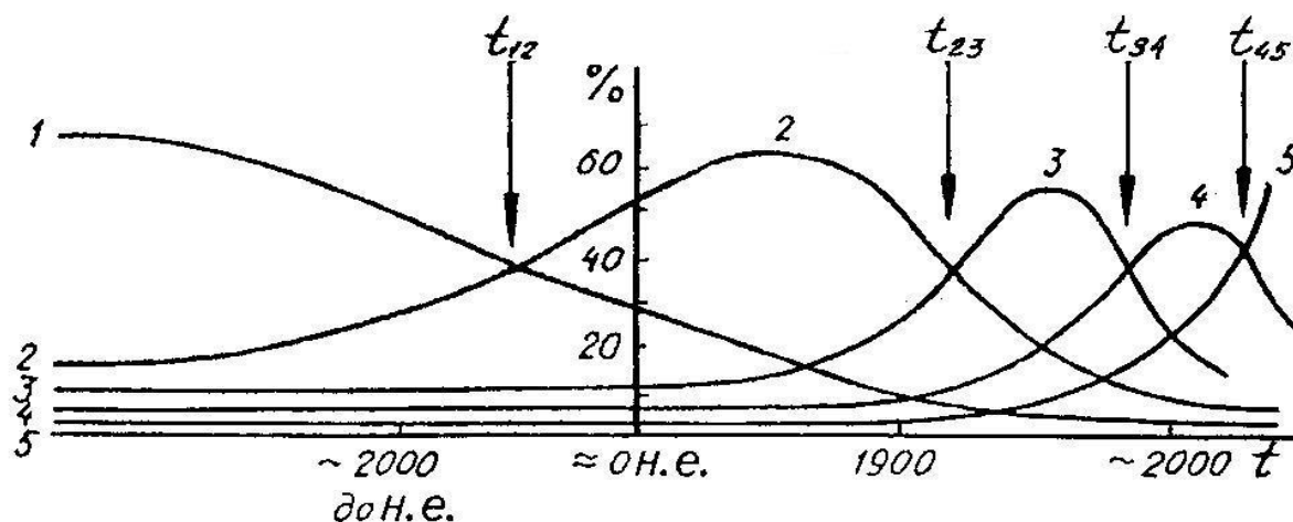
Рис.2. Схематический график эволюции структуры процессов воспроизводства элементов общества (нелинейный масштаб времени)
